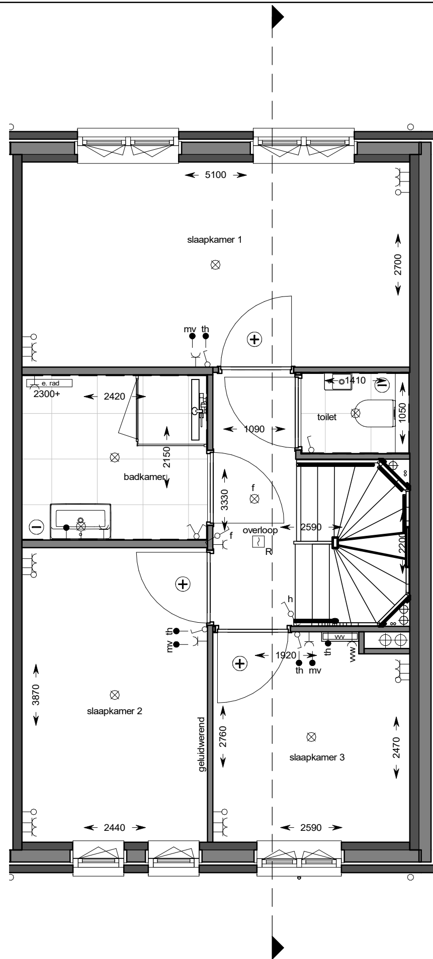
eerste verdieping
